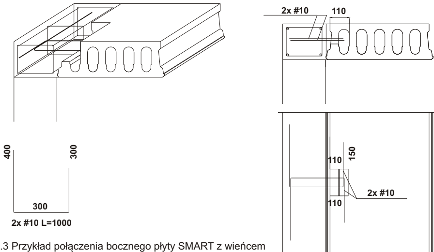
rys.3 Przykład połączenia bocznej płyty SMART z wieńcem
